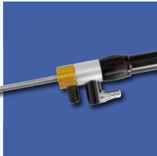
TV-Endoskop mit integriertem Mikrokameraadapter mit angewinkeltem Lichtleiteranschluß für beengte Einbauten
